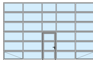
ALR F42, ALR F42 Thermo, ALR 67 Thermo Disposición central de la puerta peatonal incorporada Acristalamiento completo
